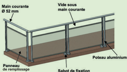
Version avec vide sous main courante
